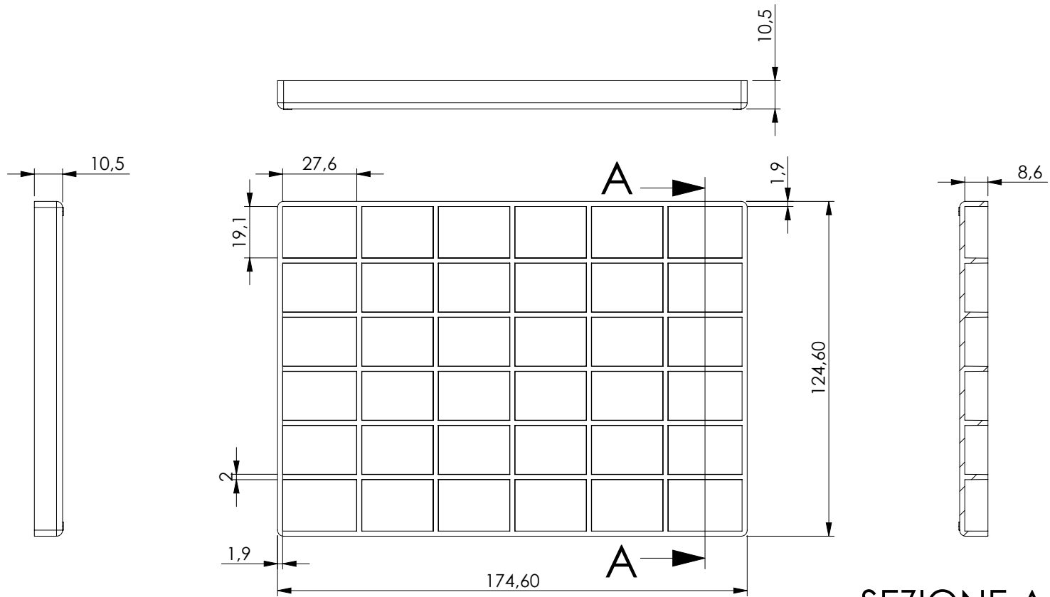
SEZIONE A-A
